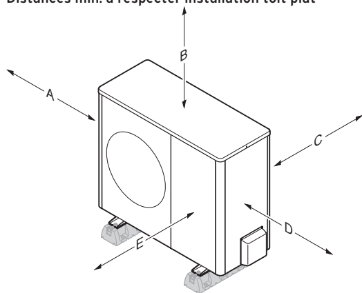
Distances min. à respecter installation toit plat
