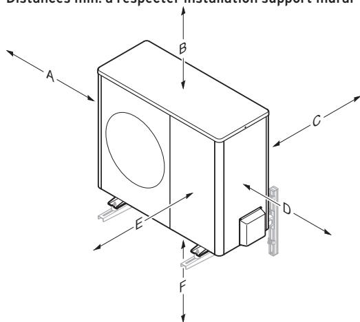
Distances min. à respecter installation support mural
