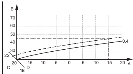
A Außentemperatur °C C Raumtemperatur °C B Vorlaufsoltemperatur °C D Achse a
